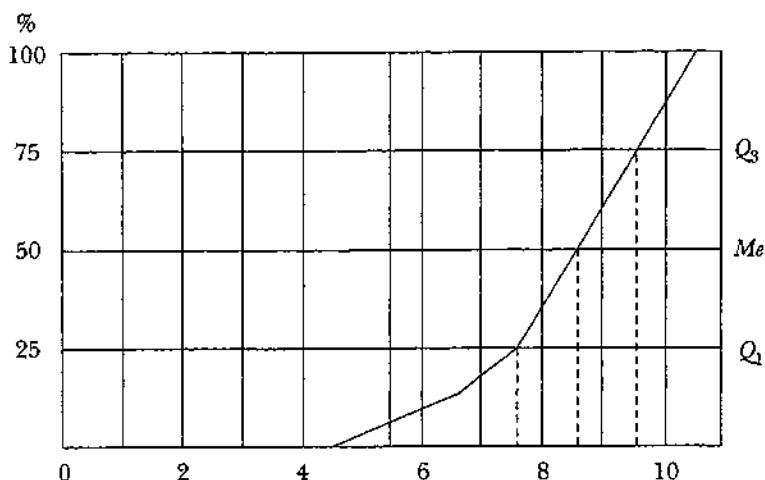
Рис. 3.4. График распределения судейских оценок для построения шкалы равных интервалов
