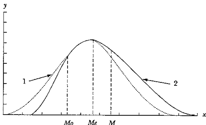
Рис. 3.5. Распределения: 1 — нормальное; 2 — скошенное
